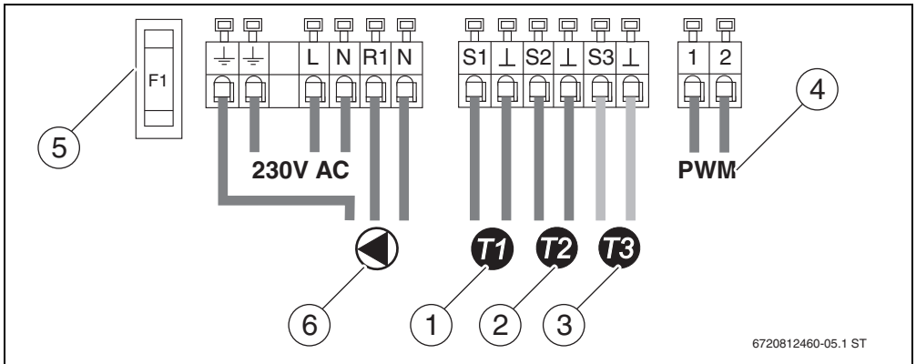
Obr. 8 Schéma pripojenia
