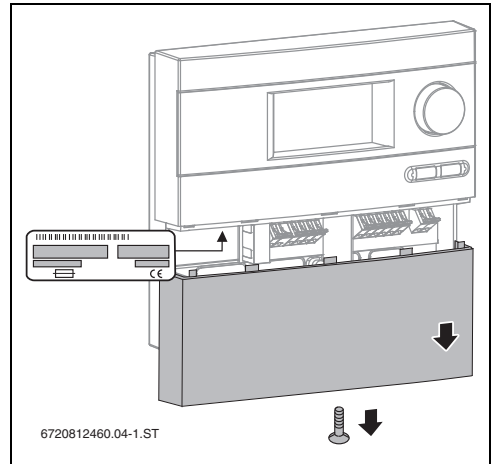
Obr. 5 Typový štítok
