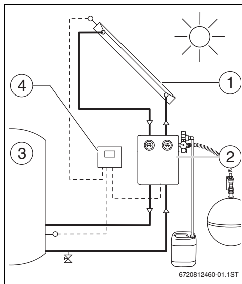
Rys. 3 Schemat instalacji
